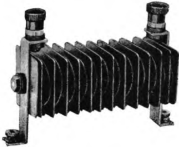
Kuprox gelijkrichter voor gloeistroom 4 Volt 1 Amp.
