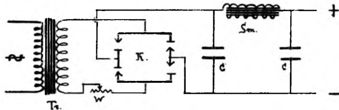
Principe-schema van den in dit artikel beschreven gelijkrichter
